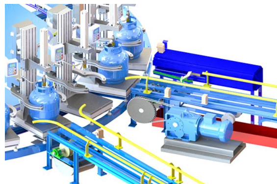
Mecanismo Ingreso / Salida Cilindros a Carrusel
