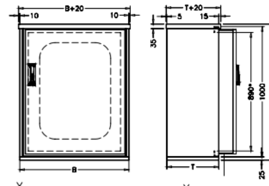
Gabinetes con / sin luna frontal
